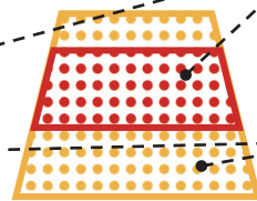
がけ崩れ
