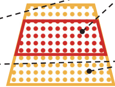
がけ崩れ
