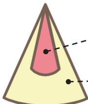
土石流
