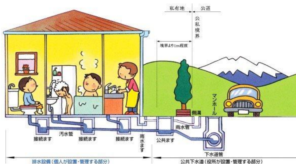
図 3-11 下水道の概要
