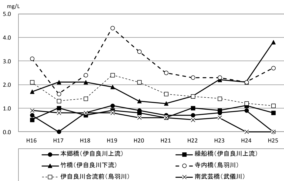
図 3-3 BOD（75%値※）の推移
