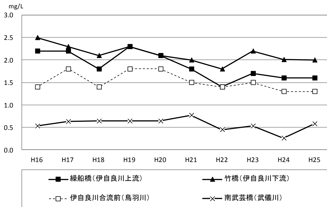
図 3-7 全窒素の推移
