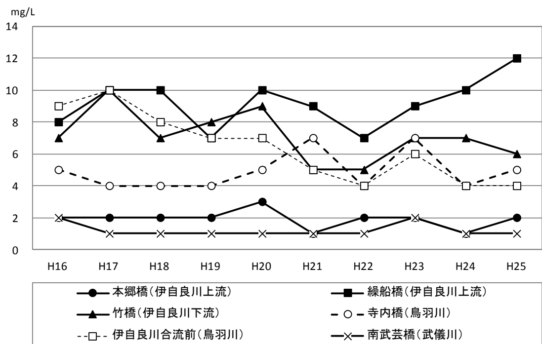
図 3-4 S Sの推移
